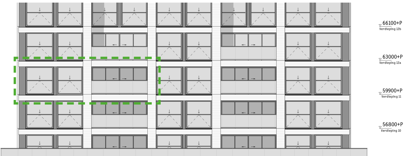
Zuidgevel
