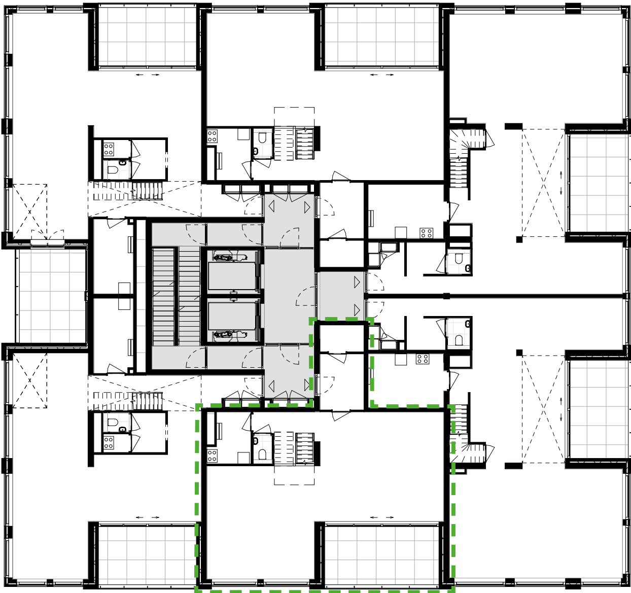
Plattegrond verdieping 12
