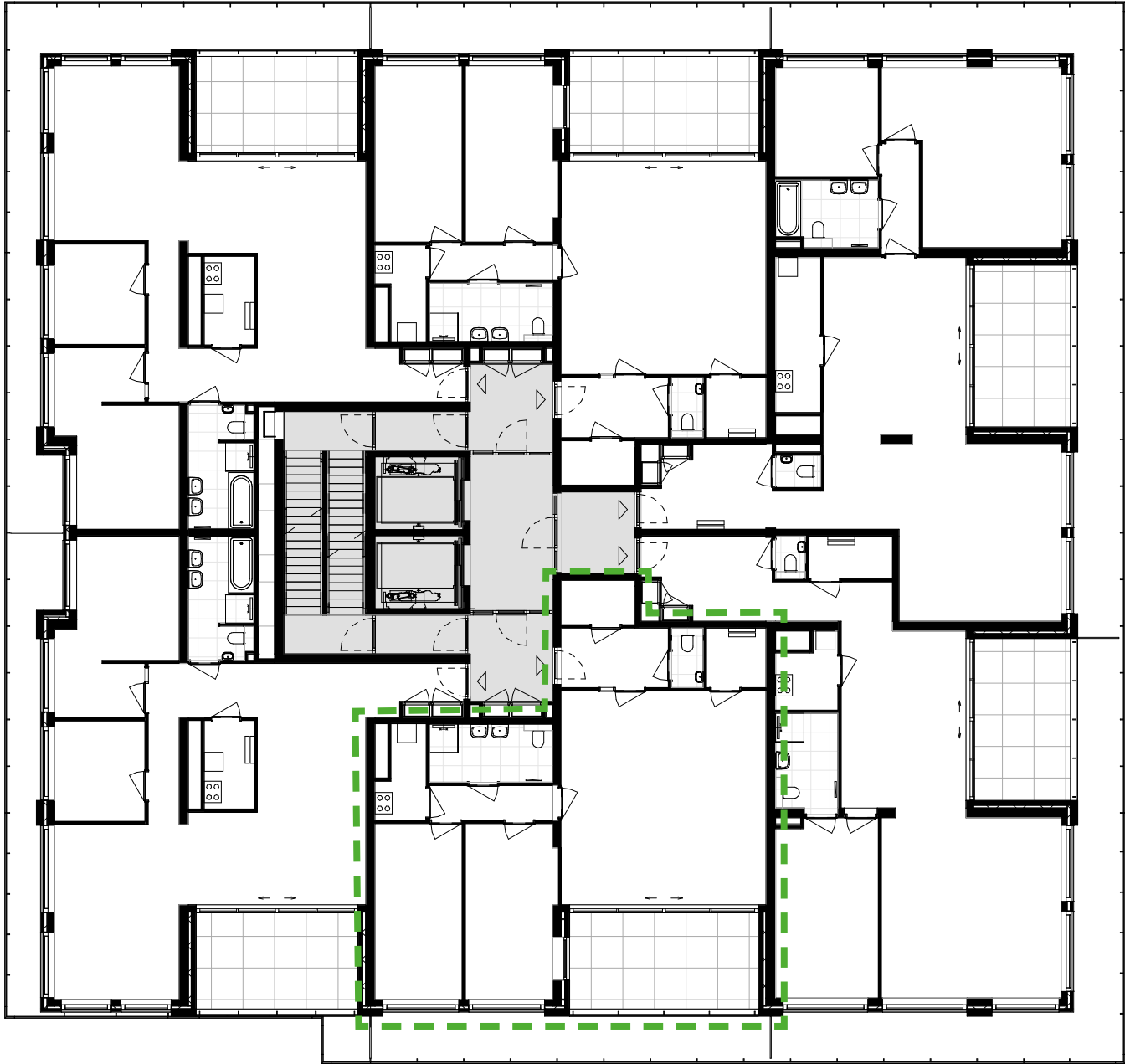
Plattegrond verdieping 10
