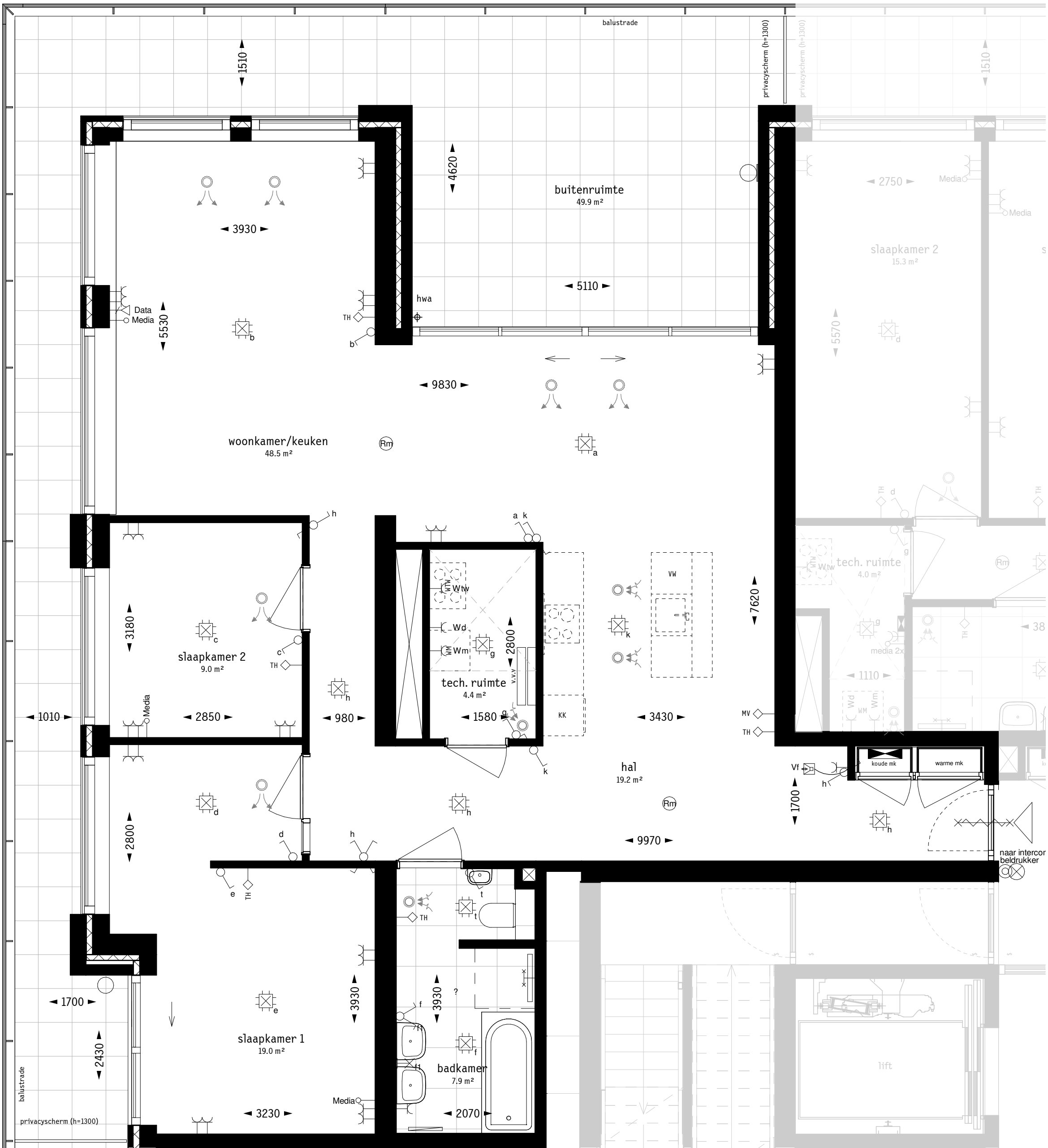
Plattegrond
